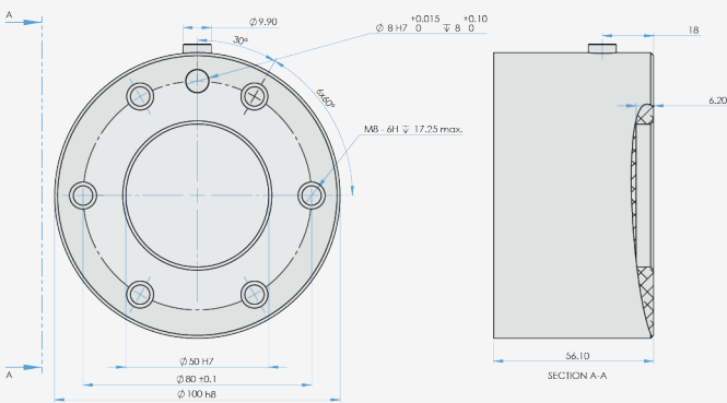
Wymiary i zasięg UR20
