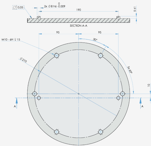
Kołnierz narzędzia do UR20
