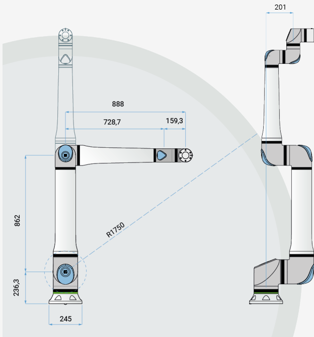
Wymiary i zasięg UR20
